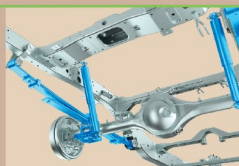
Hệ thống treo sau nhíp thiết kế mới êm dịu hơn, phù hợp sử dụng đa mục đích.
