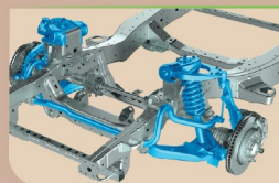
Hệ thống treo trước độc lập, tay đòn kép giúp xe êm ái và ổn định.
