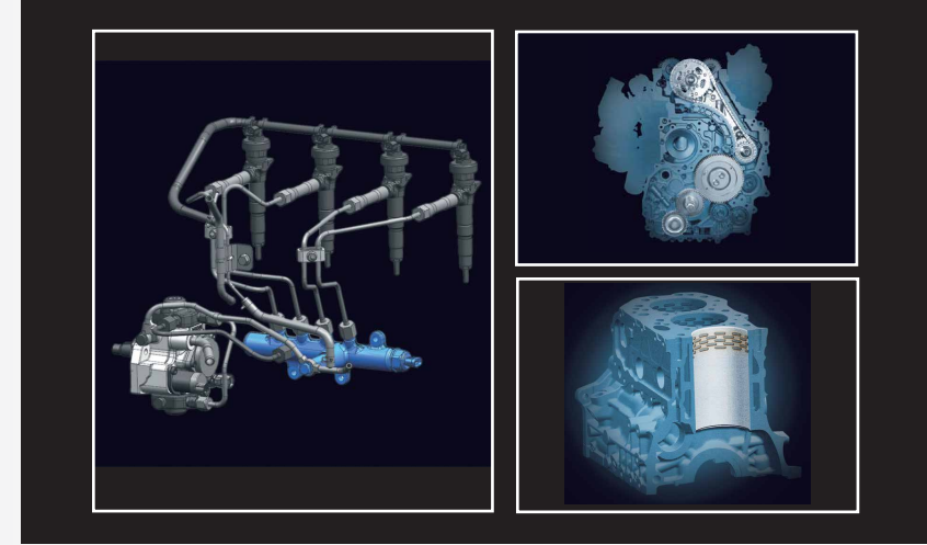
Động cơ đầu 4 xy lanh thẳng hàng, phun nhiên liệu trực tiếp sử dụng đường dẫn chung, làm mát khí nạp Diesel I4 engine, intercooler VGS turbo, common rail
